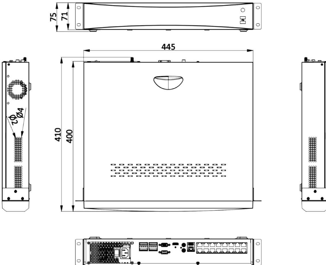
scale/1:1;Unit/mm
